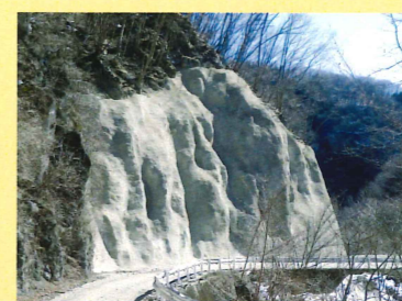
コンクリート吹付工 地山に鉄筋を組んで圧縮空気でコンクリートを吹き付けます。
