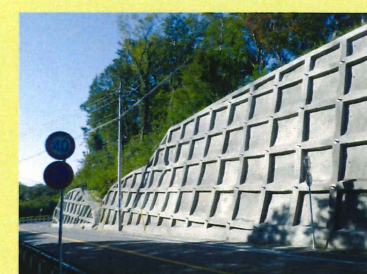
ロックボルト+法砕工 法面崩壊を抑制します。
